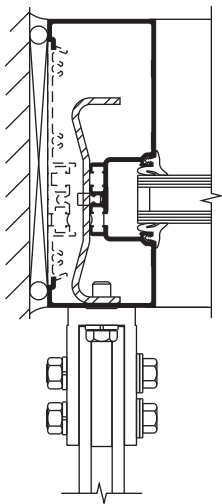
601TDE TRIFAB® JAMBA (TF 601 Y 601UT SIMILAR)
