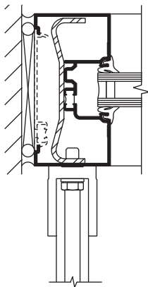
VG 451Tde TRIFAB® JAMBA (TF VG 451 Y 451UT SIMILAR)
